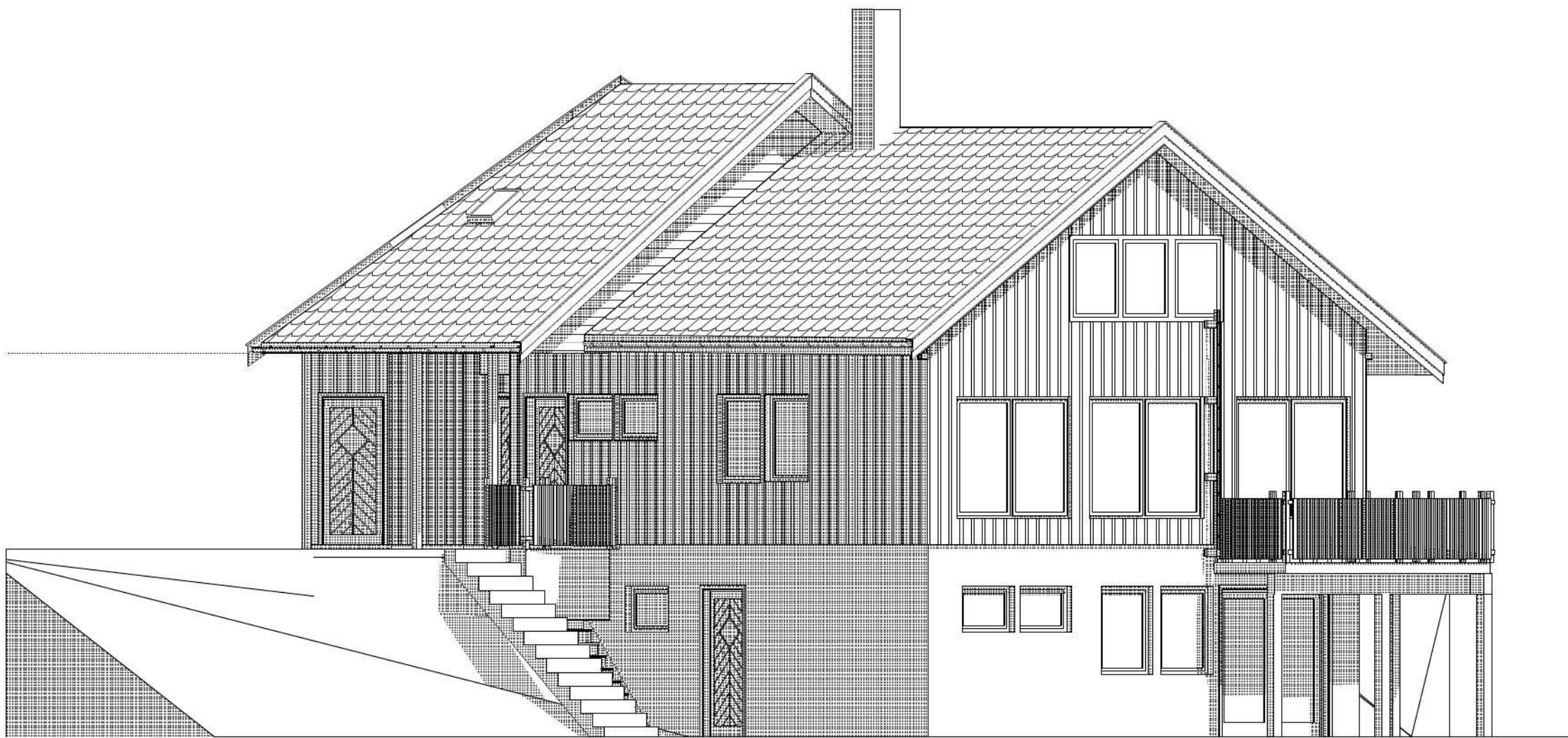
1:100 Fasade Vest
